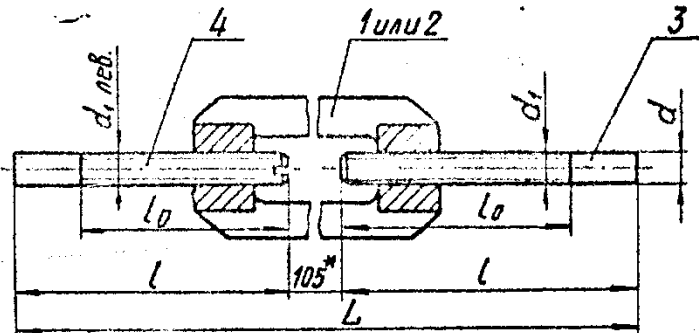
Черт. 1 Размеры в мм
